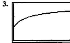
[0, 3] by [0, 3]
